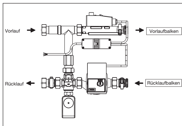
Durchflussrichtung
