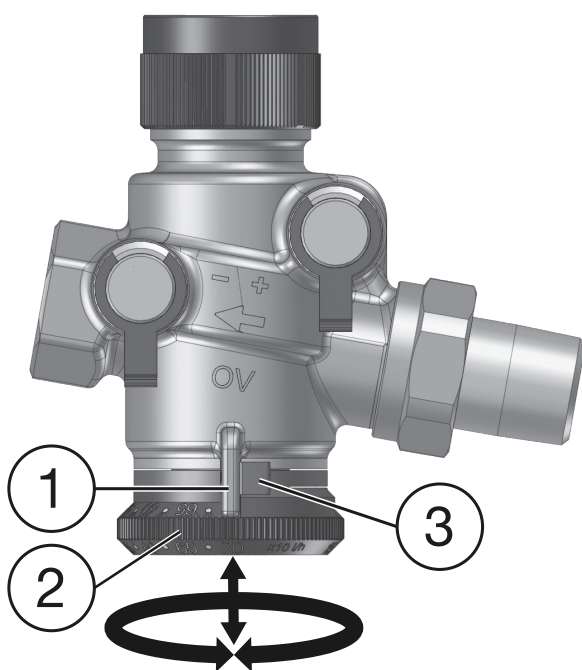
Рис. 11: Регулировка объемного потока
