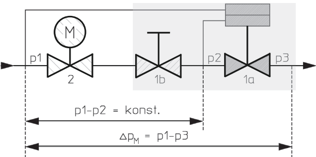
图 3: 工作原理“Cocon QTZ”，PN25
