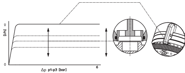
Fig. 4: Presión diferencial p1-p3 (bar)
