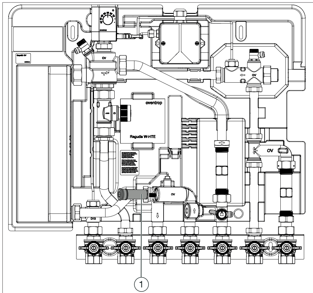
(1) Filtereinsatz / filter insert / tamis
