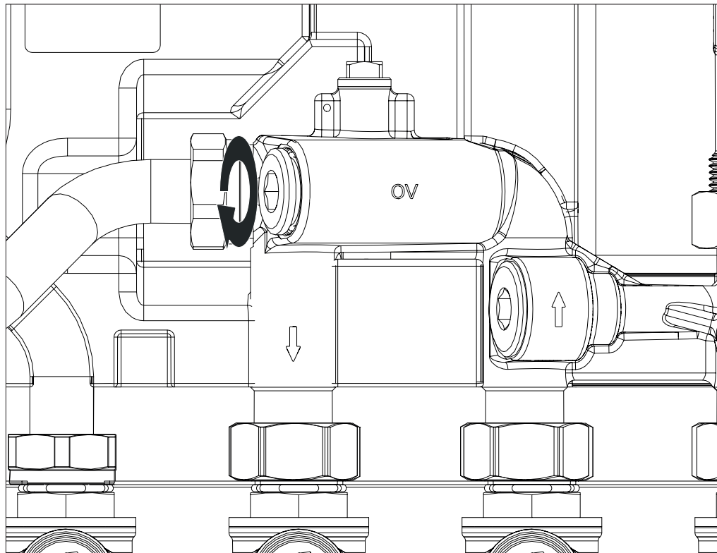
(1) Filtereinsatz / filter insert / tamis
