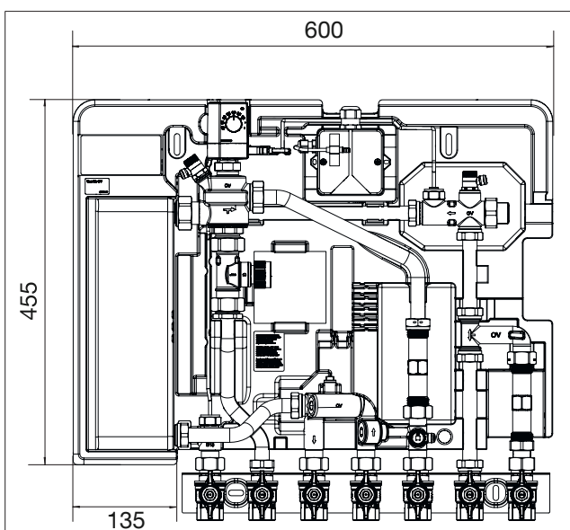
Fig. 6: Encombrements avec station d'appartement «Regudis W-HTE» en mm
