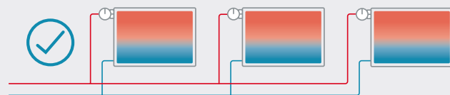
Leistungsoptimierung von Heizungsanlagen mit hydraulischem Abgleich
