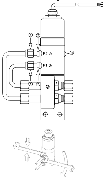
Abb. 5: Entlüftungsangabe
