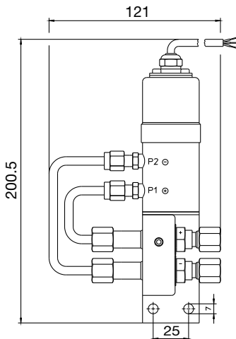
Abb. 3: Abmessungen Differenzdruckaufnehmer
