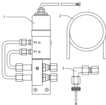
Abb. 1: Lieferumfang Differenzdruckaufnehmer
