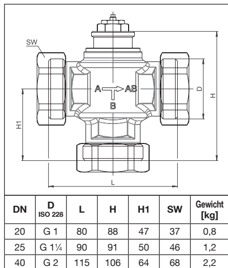
Afb. 4.1 Afmetingen
