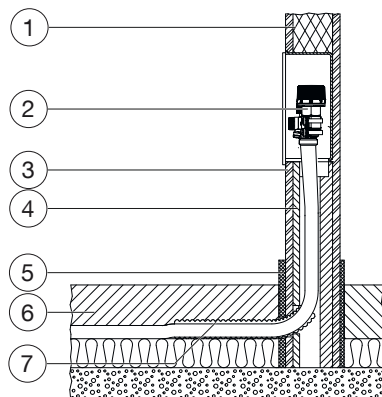
Abb. 6: Einbauquerschnitt
