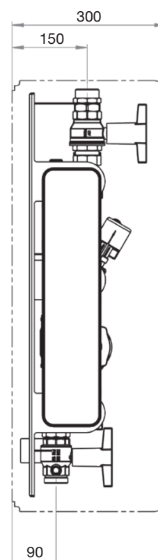
Fig. 3.9: Encombres «Regumaq X-70» (vue de côté)
