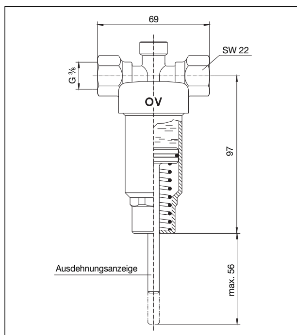
Druckausgleichsarmatur
