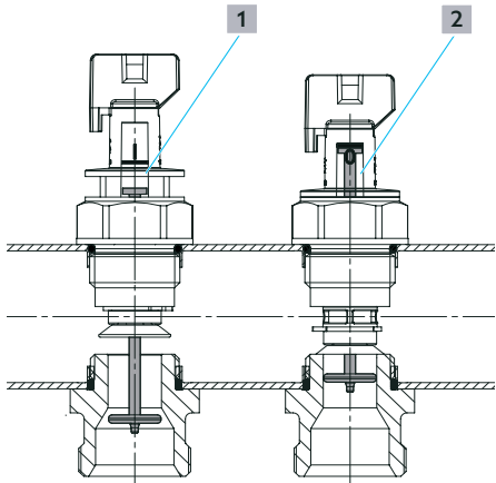
Fig. 3: Réglage de l'indicateur du débit
