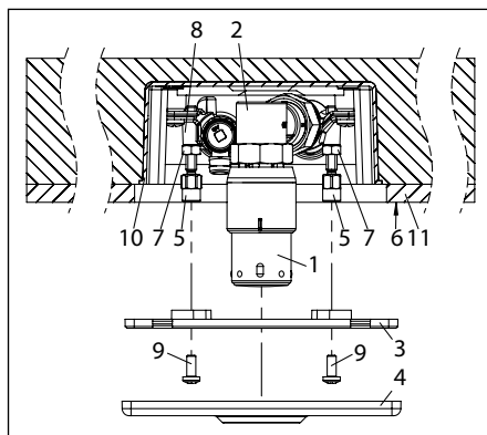
Abb. 5.4 Ausrichten Rahmenhalter
