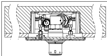
Abb. 5.5 Rahmen und Abdeckplatte montiert
