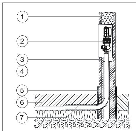
Fig. 8 : Vue en coupe de l'installation
