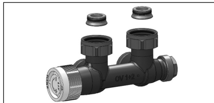
Abb. 2 Anschlussarmatur „Multiblock TU“, Eck G \frac{3}{4} ÜM x G \frac{3}{4} AG
