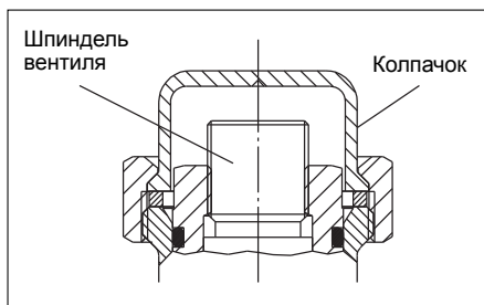
Рис. 7.1: Регулирующий вентиль
