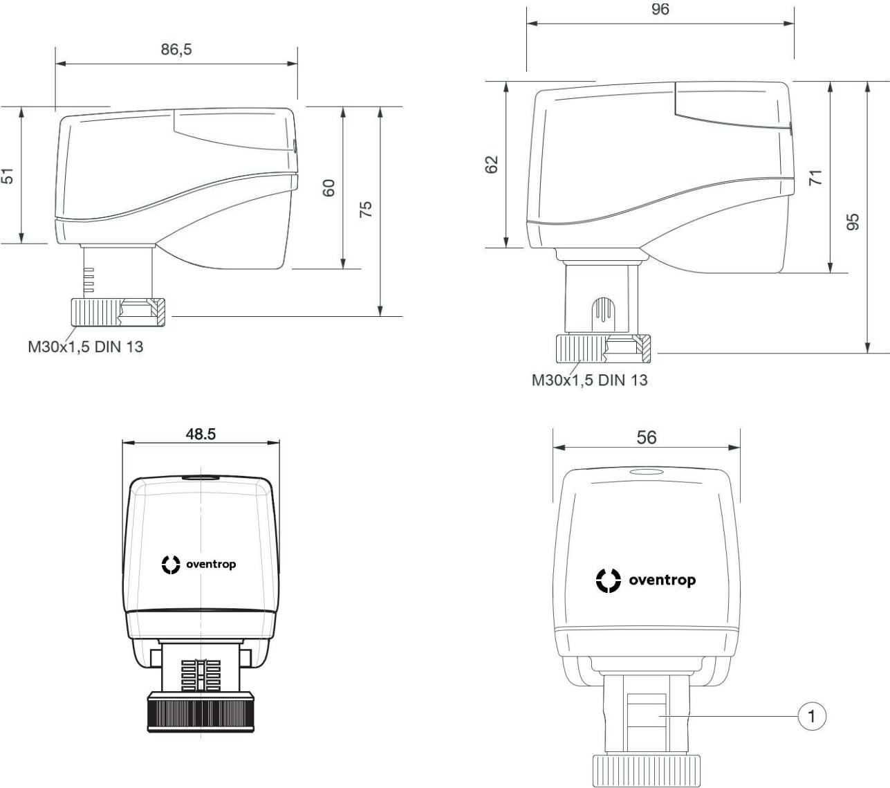
(1) Bouton-presseur pour libérer la tige de la vanne enclenchée
