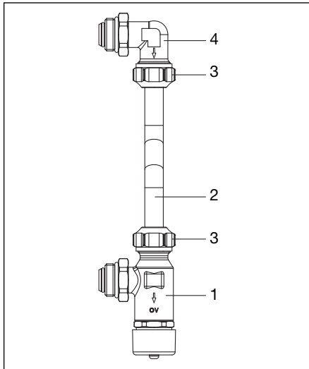
Abb. 4.1 Übersicht Überströmeinrichtung
