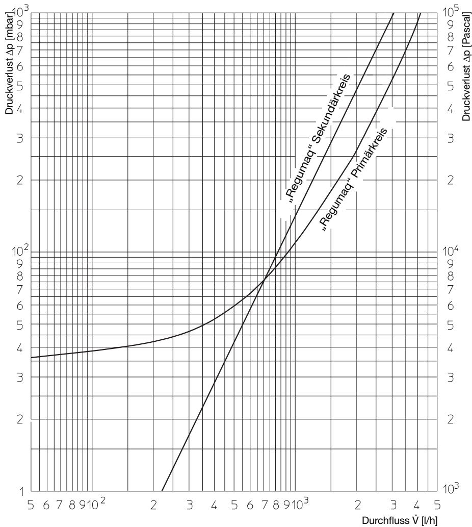
Abb. 1: Durchflusssdiagramm „Regumaq X-30-B“/„Regumaq XZ-30-B“
