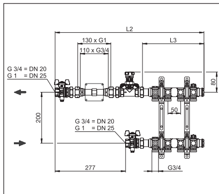
Fig. 4.2 Exemple: Jeu de raccordement no. 1 pour compteurs de calories, modèle droit, et distributeur/collecteur en acier inoxydable «Multidis SH» pour le raccordement de radiateurs, longueurs
