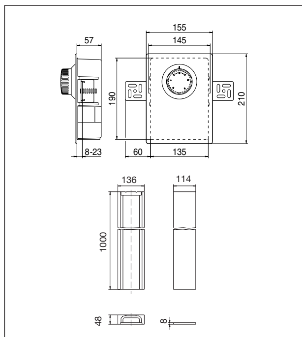
Dimensioni „Unibox E T”, „Unibox E plus” e pozzetto
