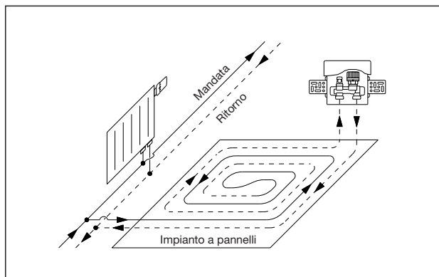
Schizzo di montaggio limitatore di temperatura del ritorno
