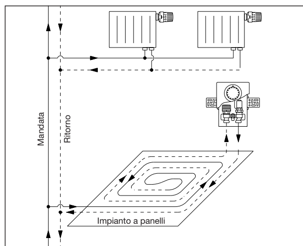
Schizzo di montaggio della regolazione della singola zona e limitatore di temperatura del ritorno
