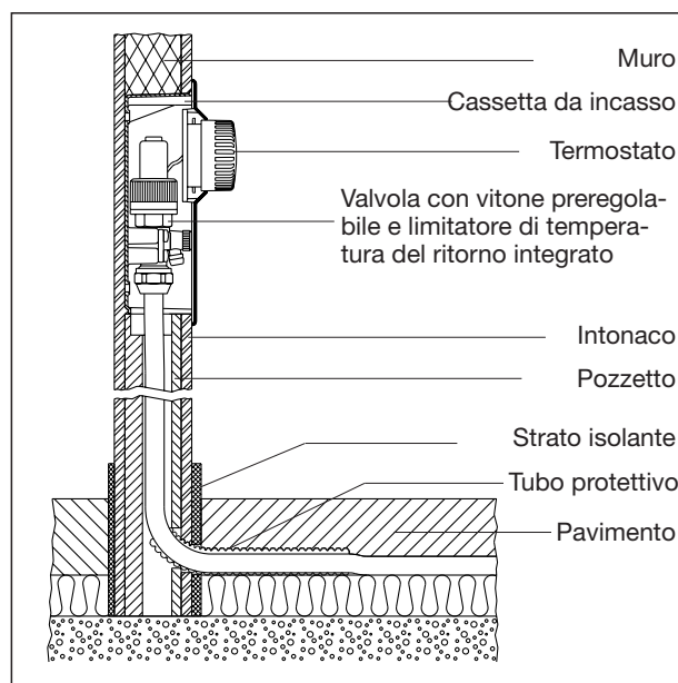
„Unibox E plus”, prof. 57 mm
