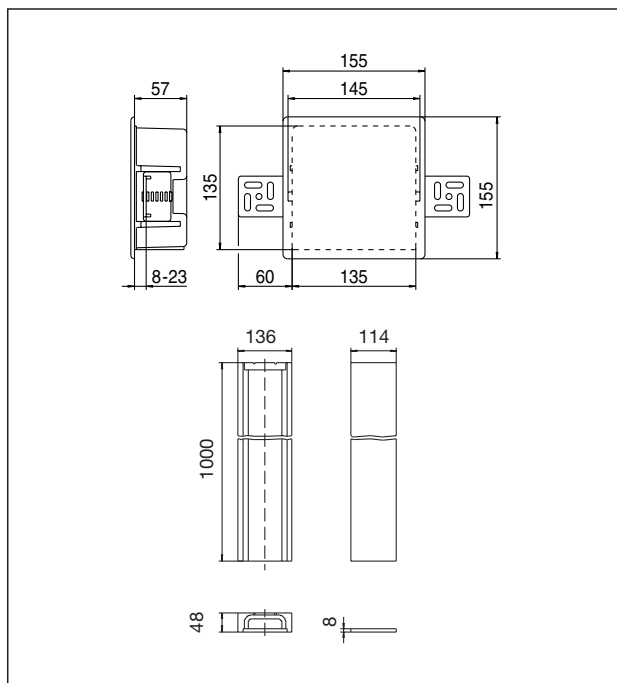
Dimensioni „Unibox E RTL” e pozzetto
