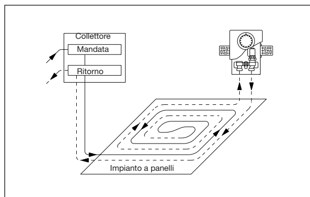
Schizzo di montaggio della regolazione del singolo ambiente
