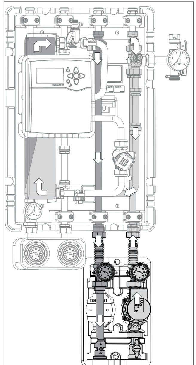
Abb. 18: Sekundärseite Regudis H-H / Regudis H-M (Beispiel Anschluss von unten)
