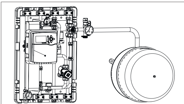
Abb. 40: Membranausdehnungsgefäß montiert
