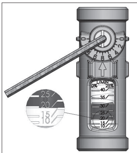
Abb. 6.3 Durchflusseinstellung
