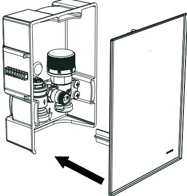
Abb. 10: Abdeckung aufsetzen
