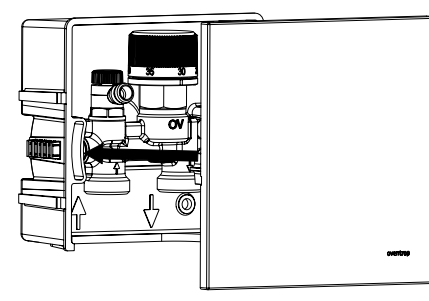
Abb. 7: Abdeckung aufsetzen
