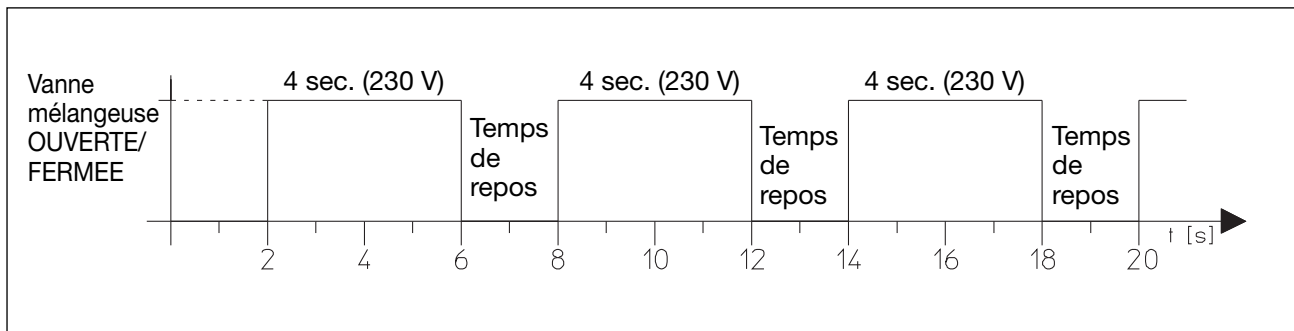
Fig. 11 Intervalle vanne mélangeuse OUVERTE/FERMEE
