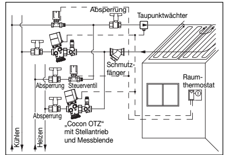
Abb. 6.2 Vierleitersystem
