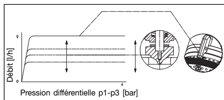
Fig. 5.6 Ligne caractéristique du débit pour préréglages différents
