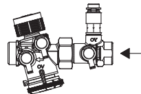
Abb. 6.3 Messblendeneinsatz wechseln
