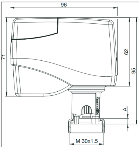
Dimensiunile actatoarelor, cod art. 1158012/13
