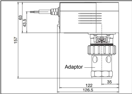
Dimensiunile actatoarelor, cod art. 1158011
