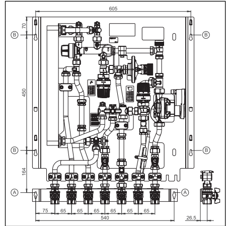
Abb. 5.5 Anschlussschema Kugelhahnanschluss- leiste 1341180
