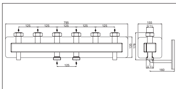
Osztó méretei DN 25, 3 kör
