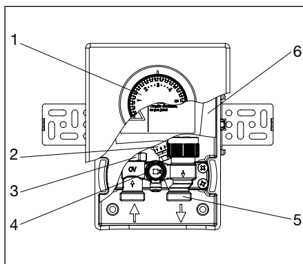
Fig. 4.1 Vue d'ensemble «Unibox E BV»
