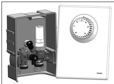
Abb. 1 „Unibox E BV“ Art.-Nr. 1022662
