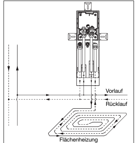
Abb. 5.5 Einbauskeizze mit „Unibox E BV“ im Montagekanal, Art.-Nr. 1022654
