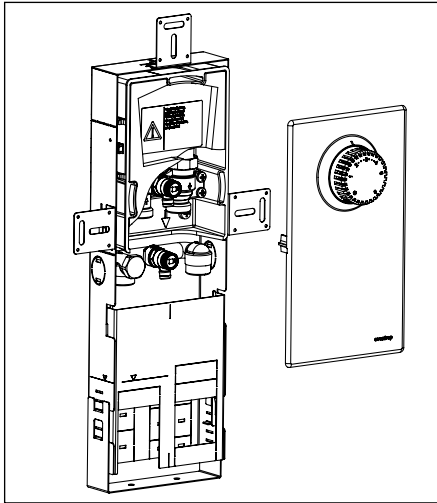
Abb. 5.4 „Unibox E BV“ im Montagekanal Art.-Nr. 1022654
