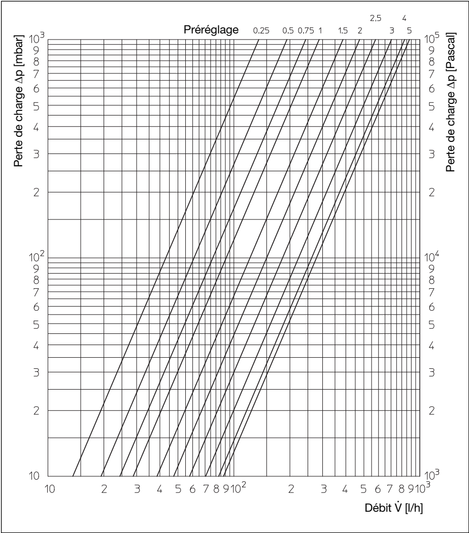
Illustr. 7.3: Diagramme mécanisme de réglage, écart P de 2 K, préréglage bypass 2,3 (75%)
