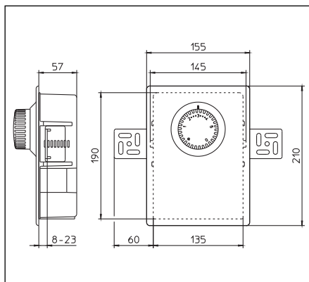
Illustr. 3.1 Encombrements «Unibox E BV»
