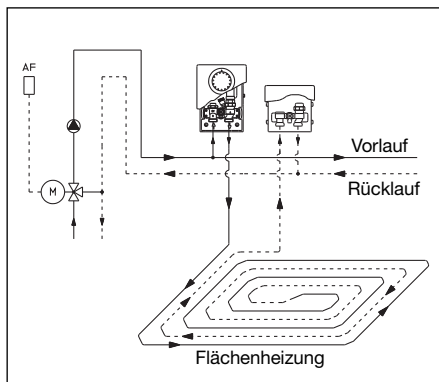
Abb. 5.3 Einbauskizze mit „Unibox RLA“ alternativ im Rücklauf
