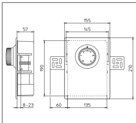
Abb. 3.1 Abmessungen „Unibox E BV“
