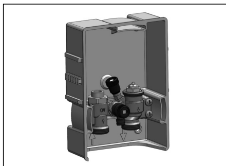
Abb. 2 „Unibox E BV“ Art.-Nr. 1022676 ohne Abdeckplatte und Thermostat für Montagekanal mit Heizkreisabsperung (Art.-Nr. 1022654)
