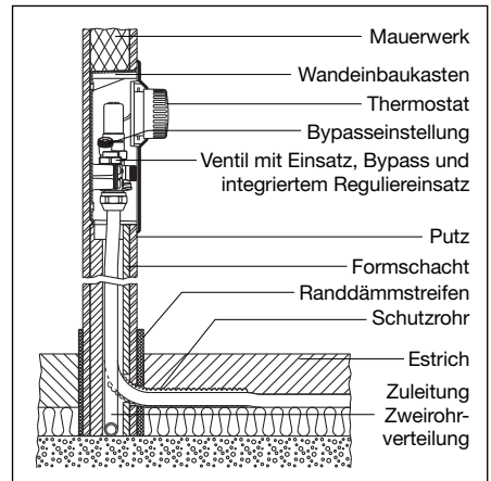
Abb. 5.1 Schnitt „Unibox E BV“ in Wand
