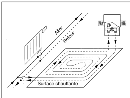
Croquis d'installation
