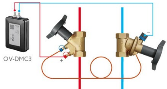
图 7： 连接图 OV-DMC3
