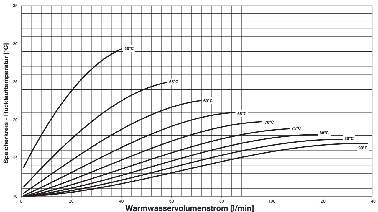
Rücklauftemperatur Speicherkreis bei unterschiedlichen Vorlauftemperaturen - Trinkwassererwärmung von 10 °C auf 50 °C -
