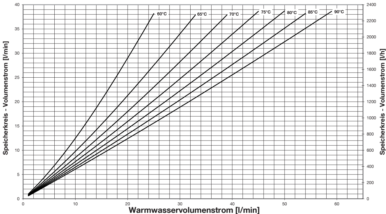
Abb. 45: Volumenstrom Speicherkreis - Trinkwassererwärmung auf 60 °C
