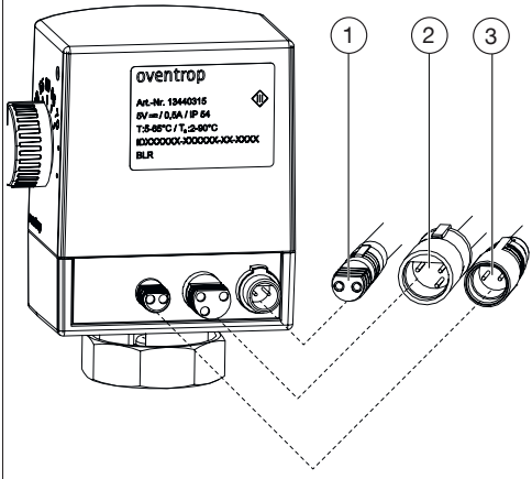
Abb. 5: Steckverbindungen
