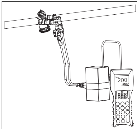
Abb. 5.5 Differenzdruckmessung
