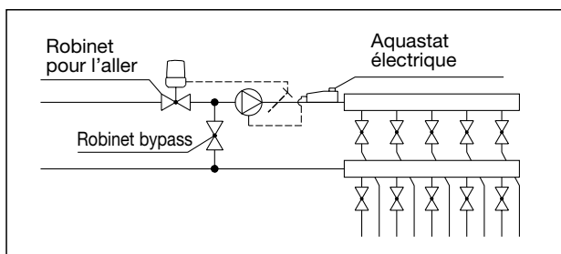
Limitation de la température de départ
