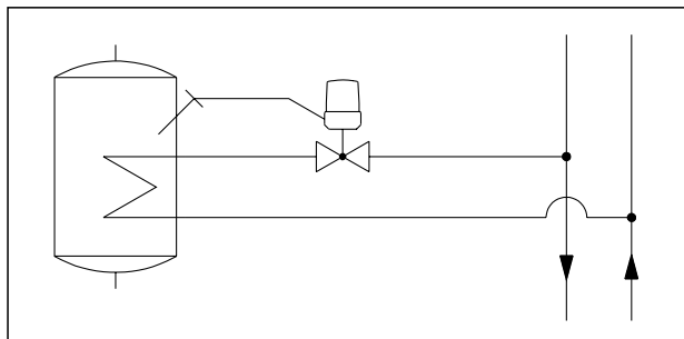
Echauffement d'eau domestique avec réservoir
