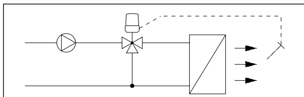
Régulation de la température dans réchauffeurs d'air
