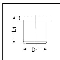
Douille à souder
