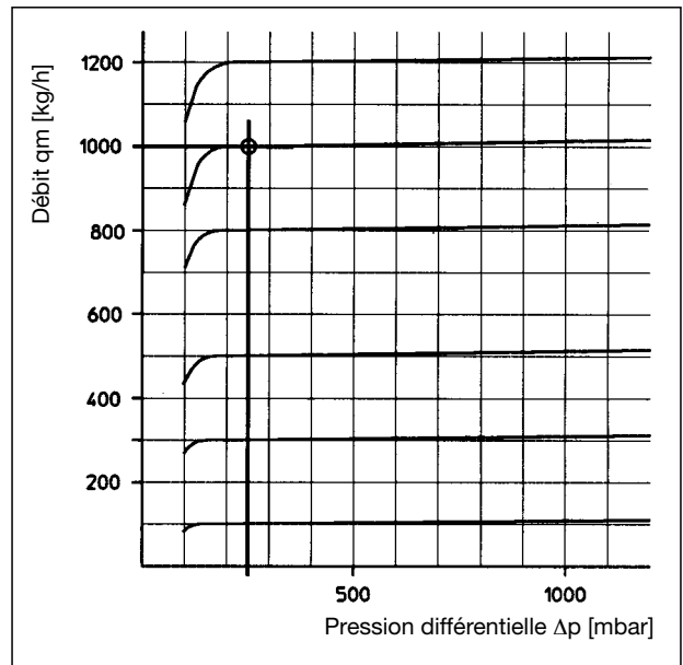
Extrait du diagramme DN 20
