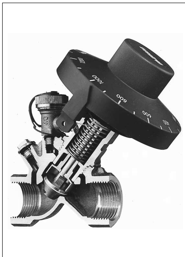
Vue en coupe
