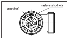
Obr.2 Přednastavení termostatického ventilu „AV9“
