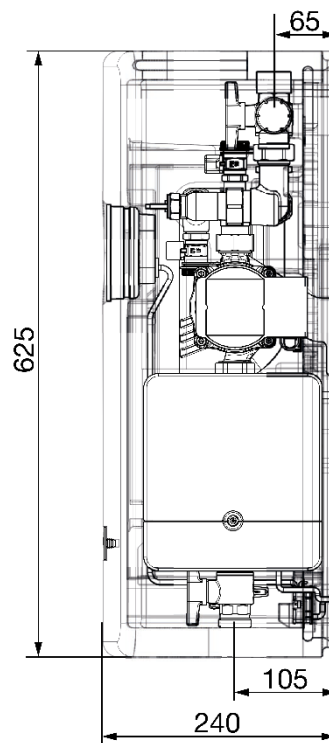
Abmessungen Regumaq X-45 (Seite)
