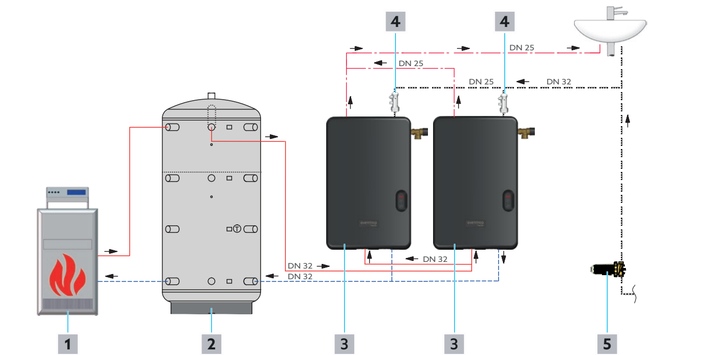
Fig. 4: Schéma d'installation avec un ballon d'eau chaude et deux stations d'eau chaude sanitaire
