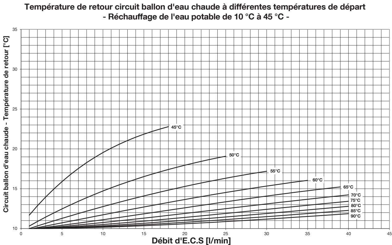
Fig. 43: Température de retour du circuit ballon d'eau chaude - Réchauffage de l'eau potable à 45 °C
