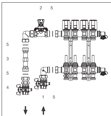
Abb. 6.1: Wärmemengenzähler-Anschluss-Set 1, Eckform, Lieferumfang und Anordnung der Komponenten bei Linksanschluss.
