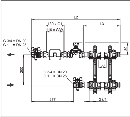
Abb. 4.2 Beispiel: Wärmemengenzähler-Anschluss-Set 1, Durchgangsform, und „Multidis SH“ Edelstahl-Verteiler für Heizkörperanbindung, Baulängen und Bautiefe
