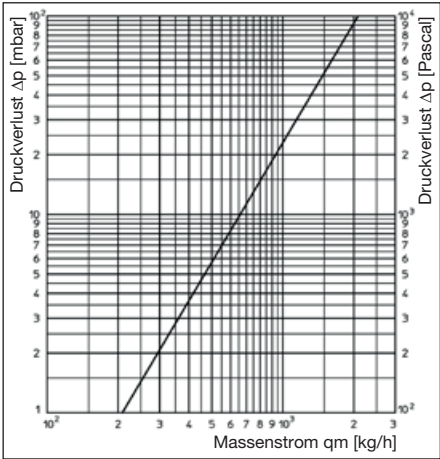
Diagramm 1: Druckverlust Wärmemengezähler Anschluss-Set 1
