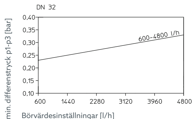
Bild 13: Min.- differensstryck
