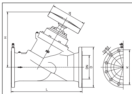
Fig. 3 Encombrements DN 200 à DN 300
