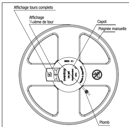
Fig. 7 Blocage de la poignée manuelle DN 200 à DN 300
