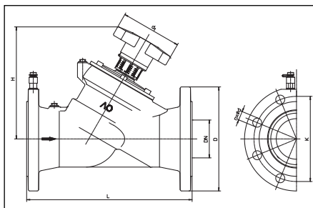
Abb. 2 Abmessungen DN 65 bis DN 150
