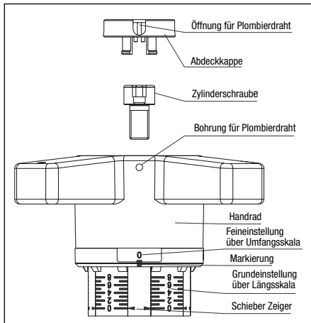
Abb. 5 Handbetätigung DN 65 bis DN 150
