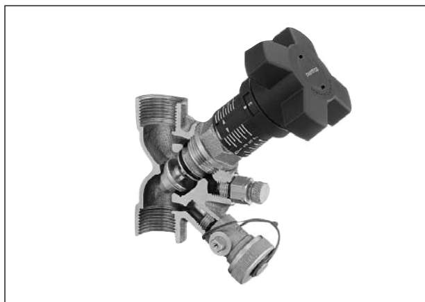
Регулирующий вентиль „Hydrocontrol” PN 16 бронзовый
