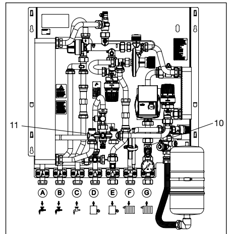
Abb. 8.1 Einbauposition Schmutzfänger
