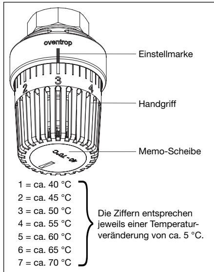
Abb. 8.4 Einstellung Trinkwassertemperatur
