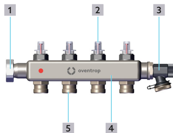
Fig. 1: Construction du distributeur pour l'aller
