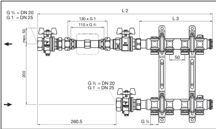
Abb. 3 Wärmemengenzähler-Anschluss-Set, Durch-gangsform, und „Multidis SH“ Edelstahl-Verteiler für Heizkörperanbindung, Baulängen
