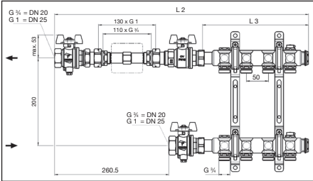
Fig. 3 Jeu de raccordement pour compteurs de calories, modèle droit, et distributeur/collecteur en acier inoxydable «Multidis SH» pour le raccordement de radiateurs, longueurs
