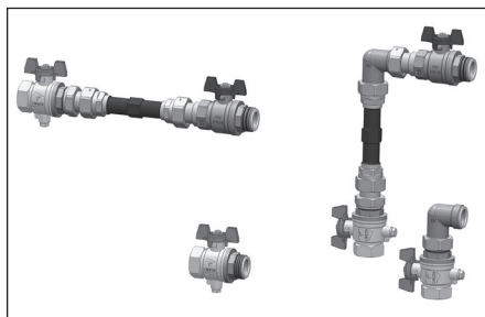
Abb. 1 Wärmemengenzähler-Anschluss-Set, Durchgangs- und Eckausführung
