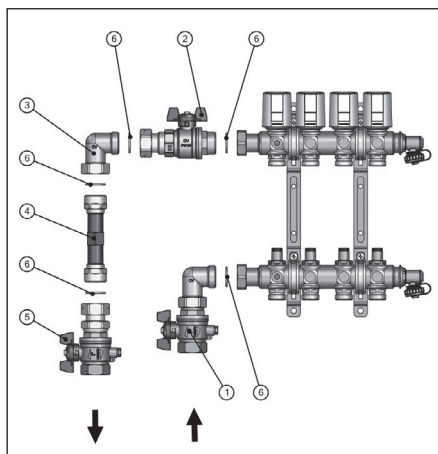
Fig. 4: Jeu pour le raccordement de compteurs de calories, modèle équerre, fourniture et placement des composants pour raccordement à gauche
