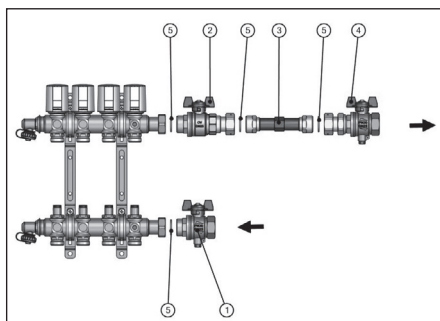
Fig. 5: Jeu pour le raccordement de compteurs de calories, modèle équerre, fourniture et placement des composants pour raccordement à droite
