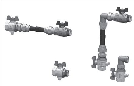
Fig. 1 Jeu de raccordement pour compteurs de calories, modèle droit et équerre
