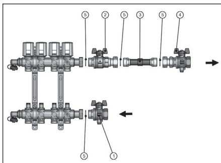
Abb. 5: Wärmemengenzähler-Anschluss-Set, Durchgangsform, Lieferumfang und Anordnung der Komponenten bei Rechtsanschluss
