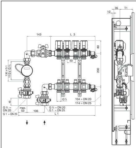
Abb. 2 Beispiel: Wärmemengenzähler-Anschluss-Set, Eckform und „Multidis SFQ“ Edelstahl-Verteiler für Flächenheizung und -kühlung, Baulängen und Bautiefe
