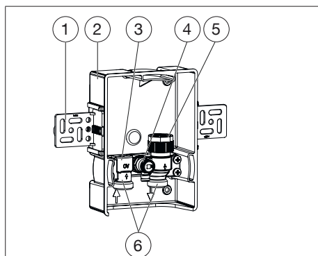
Abb. 2: Aufbau „Unibox T vario“
