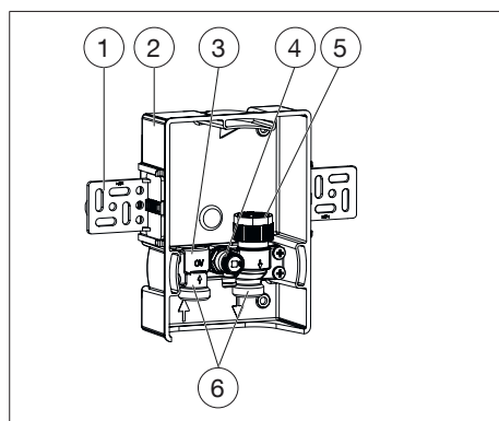
Fig. 2: Configuration de l'« Unibox T vario »
