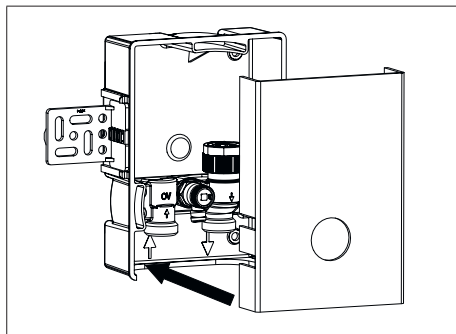
Abb. 7: Bauabdeckung aufsetzen
