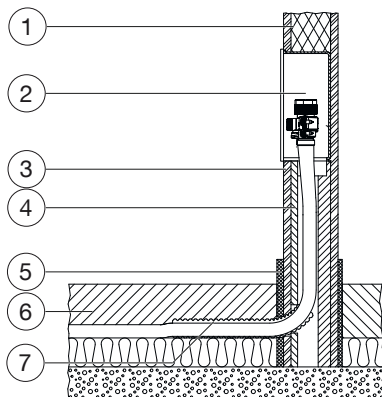
Fig. 4: Vue en coupe de l'installation
