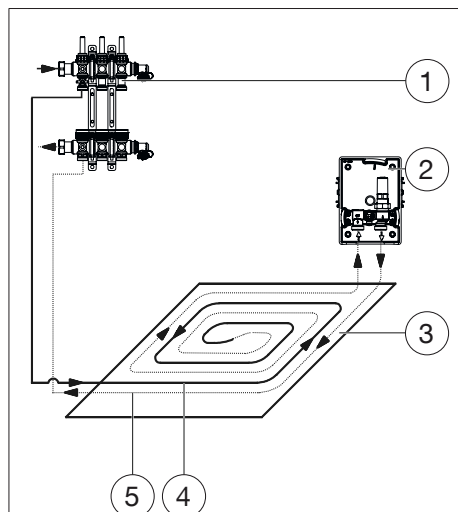
Abb. 5: Anschluss (Beispiel Betrieb mit Stellkolben)
