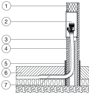
Abb. 4: Einbauquerschnitt
