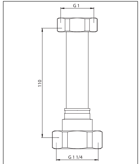
Anschlussverrohrung
