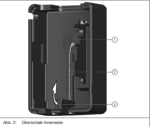
Abb. 2: Oberschale Innenseite
