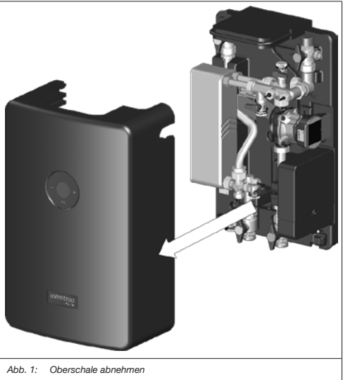
Abb. 1: Oberschale abnehmen
